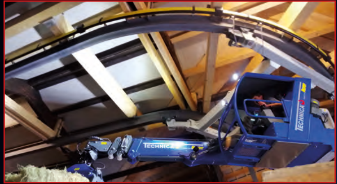
Kurvenfahrwerke sind optimale Lösungen für querliegende Gebäude (hydr. Vorsteuerung mit H/S-Ventil).
